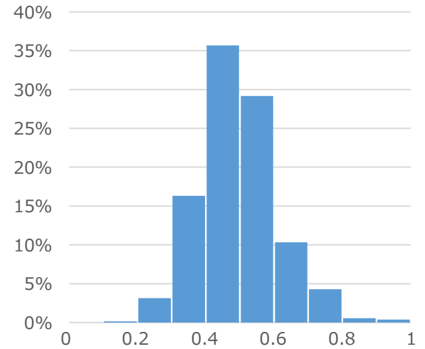
Fsp3
