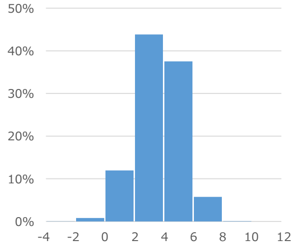
SlogP
