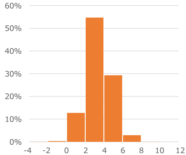
SlogP
