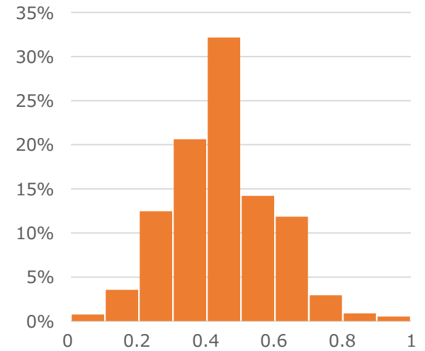
Fsp3
