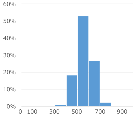
MW
