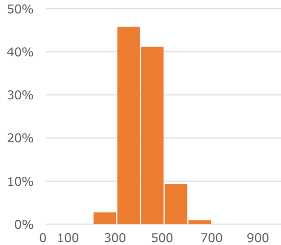
MW
